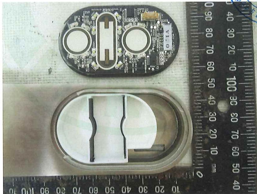
控制面板內部
